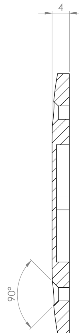
PRZEKRÓJ A-A SKALA 2 : 1
